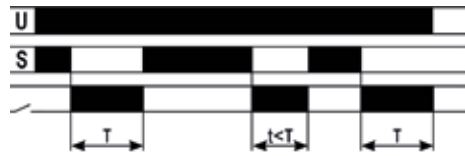
FZ74: Ausschalt-Schleiferfunktion
