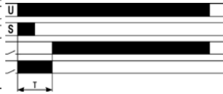
FZ77: Anzugsverz¼gert mit fester Impulszeit
