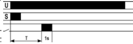
FZ77: Anzugsverz¼gert mit fester Impulszeit
