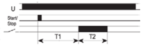
FZ41: Impulsgeber mit Start/Stop-Taste
