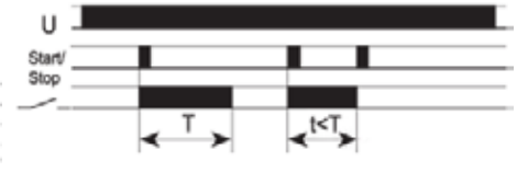
FZ38: anzugsverzögert mit Start/Stop-Taste
