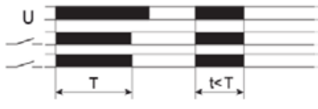
FZ19: Einschaltwischer mit Sofortkontakt
