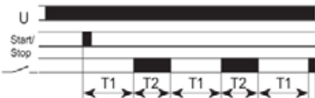
FZ40: Relé de impulso, partiendo con pausa, con contacto START/STOP
