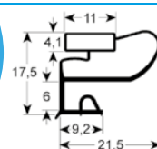
Guarnizioni mezzo bordo con magnete
