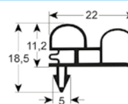
Guarnizioni ad incastro senza magnete
