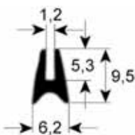
perfil 1530
