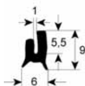
perfil 1510
