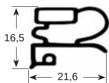
Cod. perfil 9030
