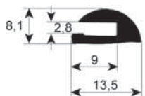
perfil 1882
