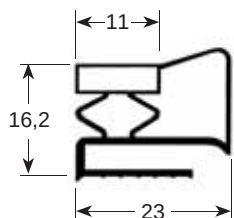
Cod. perfil 9953
