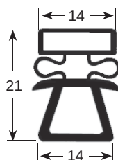
Cod. perfil 9162
