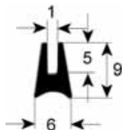
perfil 1515
