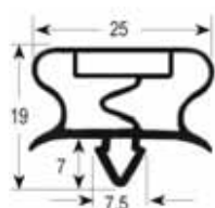
perfil 9195
