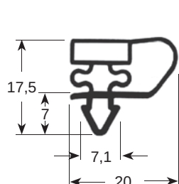
Cod. perfil 9153
