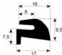
perfil 1890
