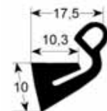
perfil 2970
