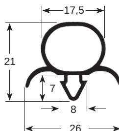
9192
