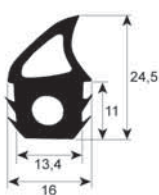
perfil 2746
