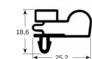
Cod. perfil 9010
