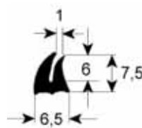
perfil 1540
