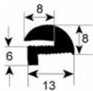
perfil 1889
