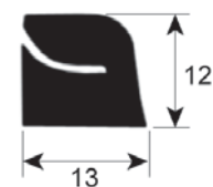
perfil 1893
