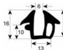
perfil 1810
