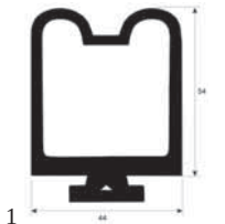
perfil 9984
