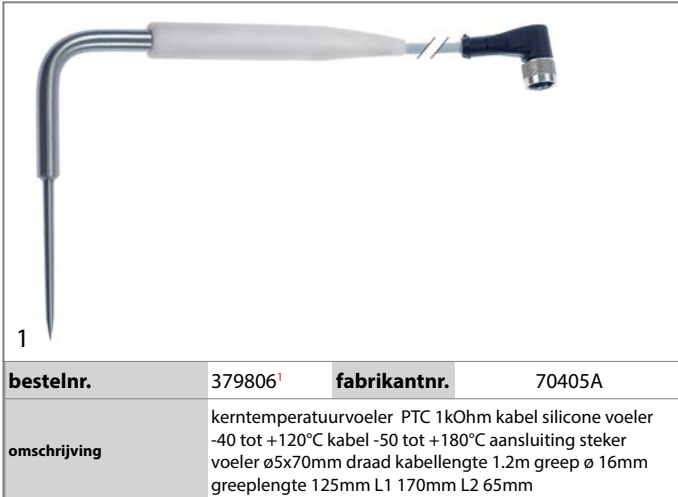
1 meerpuntvoeler
