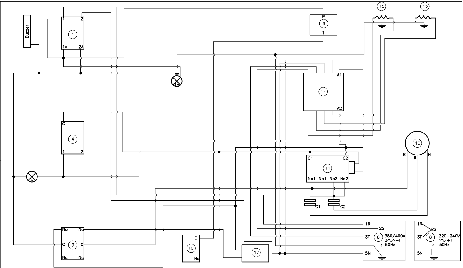
SCHEMA ELETTRICO -BISTROT 364 2005
