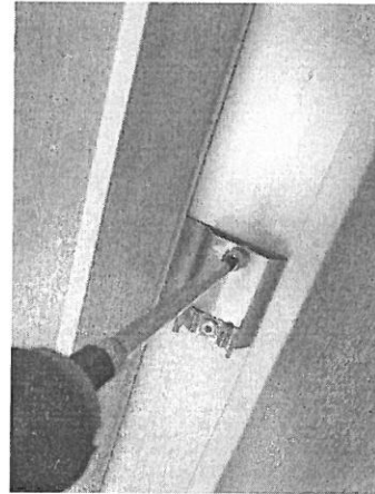
Tighten both led holders approximately 25cm from the left & right side / Σφίξτε και τα δύο μεταλλικά στηρίγματα περίπου 25 εκατοστά από την δεξιά και αριστερή πλευρά
