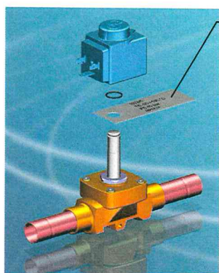
Fig.2 nuova bobina “FAST LOCK”
