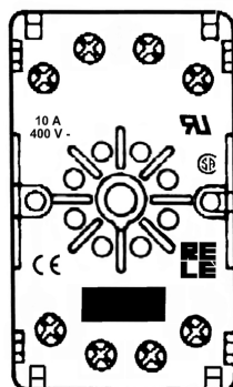
ZVE8 (8-pin)
