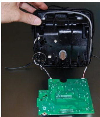
DIE HALTERUNG DER LEITERPLATTE EINSETZEN
