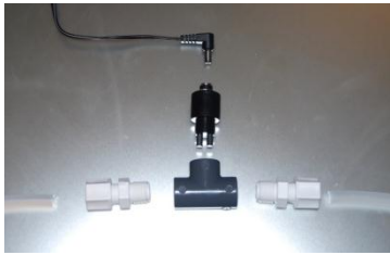
MONTAJE Y CONEXIÓN DEL EMPALME EN T CON EL TUBO DE ASPIRACIÓN SALMUERA Y LA CELDA DE TITANIO DEL GENERADOR DE CLORO...
