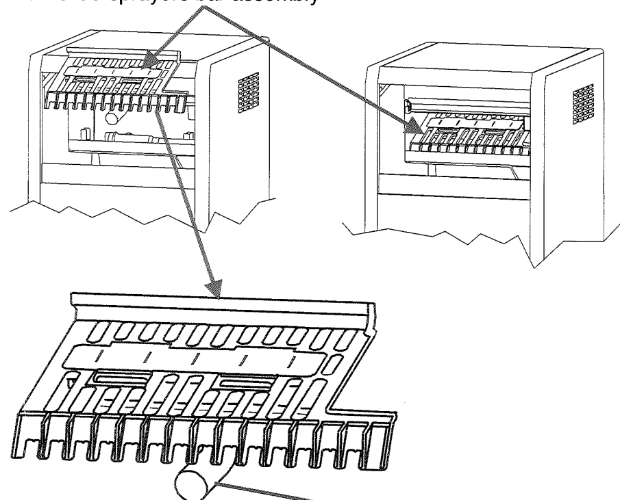
Nuovo assieme scivolo-rampa Spruzzatori / New slide-sprayers bar Assembly cod. C10626
