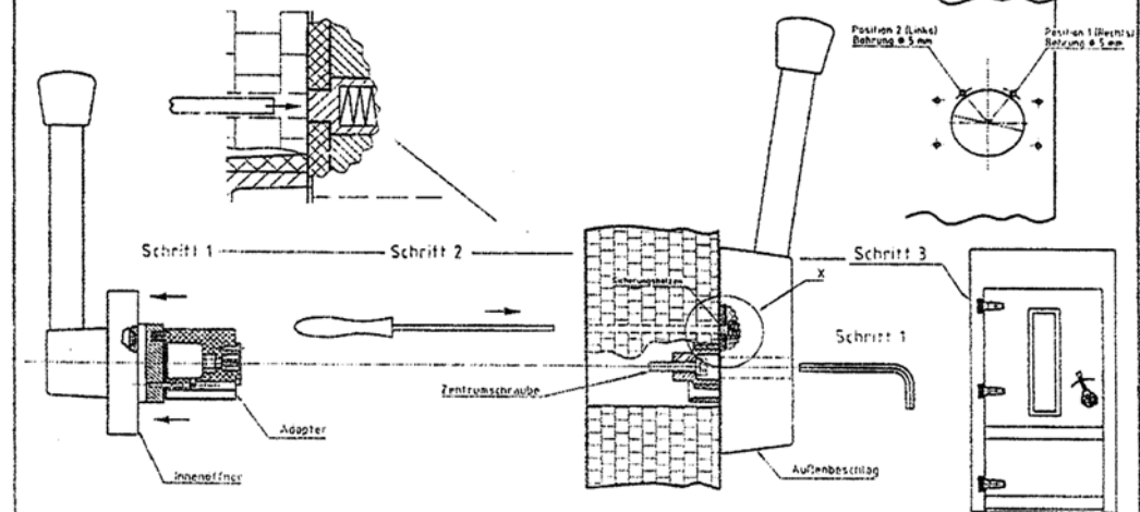
Ansicht X
