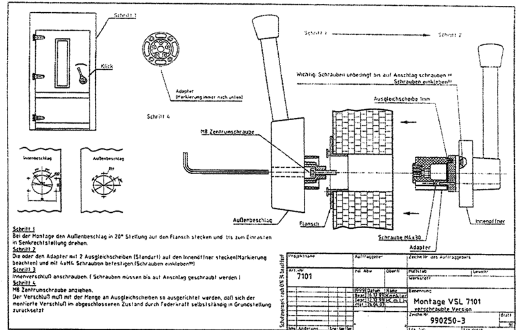
Ansicht X
