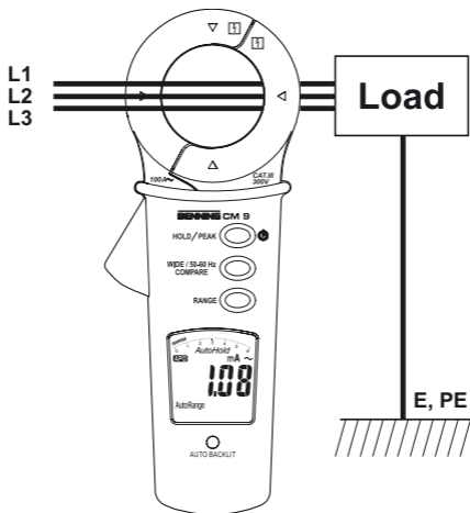
Bild 5: Differenzstrommessung, Verbraucher 3-phasig gespeist, ohne N-Leiter Fig. 5: Leakage current measurement, load supplied in three-phase, without N-type conductor Fig. 5: Mesure du courant de fuite, appareil connecté avec alimentation triphasée, sans conducteur type N Fig. 5: Medida de corriente de fugas, cargas alimentadas en trifásica sin conductor neutro Obr. 5: Svodový proud měření, spotřebič napájen 3-fázovým proudem, bez vodiče N εικόνα 5: Μέτρηση του ρεύματος διαφυγής, Τροφοδοσία καταναλωτή με 3-φασικό ρεύμα, χωρίς ουδέτερο (N) αγωγό 5. bra: Levezetési áram mérése, fogyasztó 3 fázisúan betáplálva, N-vezeték nélkül Ill. 5: Misurazione della corrente di dispersione, utenti alimentazione trifase, senza conduttore N Fig. 5: Lekstroommeting verbruikers 3-fase gevoed, zonder nul Rys. 5: Pomiar prądu upływu w sieci trójfazowej bez przewodu N См. рис. 5: Измерение тока утечки, трехфазное питание потребителя, без нейтральной Resim 5: Deşarj akımı ölçümü, tüketici 3 faz beslemeli, N kabloşuz
