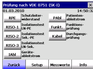
Menü, VDE 0751 SK I
