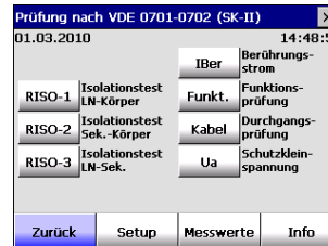
Menü, VDE 0701-0702 SK II
