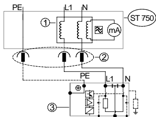
Schutzleiterstrommessung / Differenzstromverfahren: DIN VDE 0701-0702 (Sk I-II)
