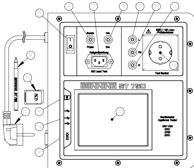
Ansicht Anschlussseite:
