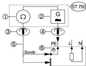
Schutzleiterprüfung R_{PE} :
