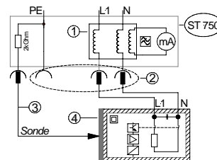
Berührungstrommessung: DIN VDE 0701-0702 (Sk I-II)
