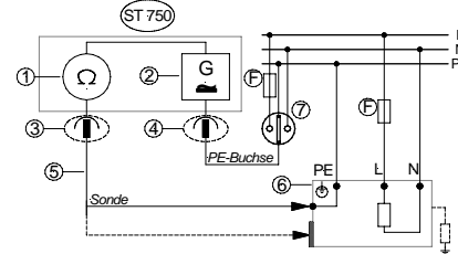
Schutzleiterprüfung R_{PE} : DIN VDE 0751-1 (SK I)
