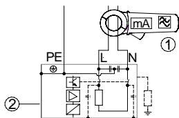
Schutzleiterstrommessung / Differenzstromverfahren: DIN VDE 0701-0702 (Sk I-II)
