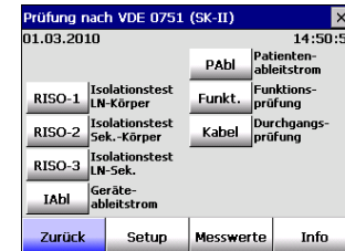
Menü, VDE 0751 SK II
