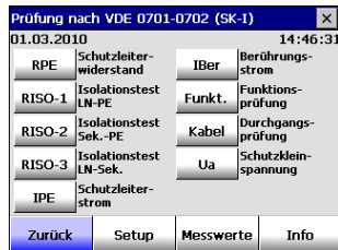
Menü, VDE 0701-0702 SK I
