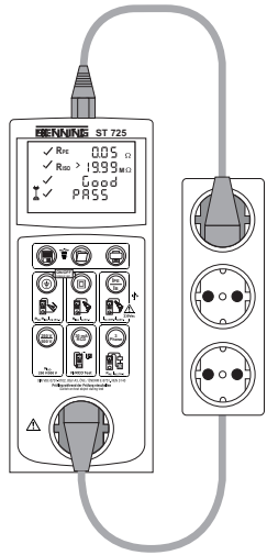
Bild 6b: Prüfung von Leitungen, Mehrfachverteilern und Leitungsroller Fig. 6b: Testing of lines, multiple distributors and cable reels Fig. 6b: Contrôle de câbles, de câbles de distribution multiple et d'enrouleurs de câble
