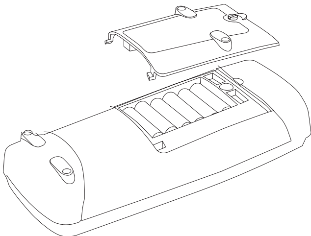
Bild 9: Batterie-/ Sicherungswechsel Fig. 9: Battery/ fuse replacement Fig. 9: Remplacement des piles/ fusibles
