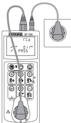
Bild 8b: Prüfung mobiler FI/PRCD Schutzschalter ( I_{\Delta N} 30 mA) Fig. 8b: Testing of portable PRCDs ( I_{\Delta N} 30 mA) Fig. 8b: Contrôle de dispositifs différentiels portatifs « PRCD » ( I_{\Delta N} 30 mA)
